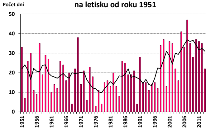
Počet dusných dní ( e \geq 18.8 hPa) v Košiciach na letisku od roku 1951
