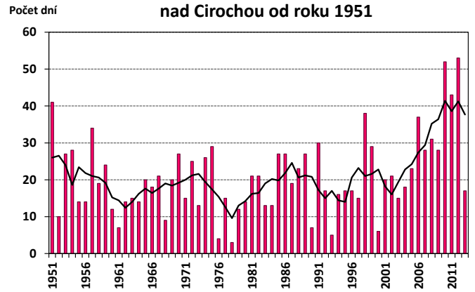
Počet dusných dní ( e \geq 18.8 hPa) v Kamenici nad Cirochou od roku 1951
