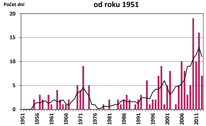
Počet dusných dní ( e \geq 18.8 hPa) v Poprade od roku 1951
