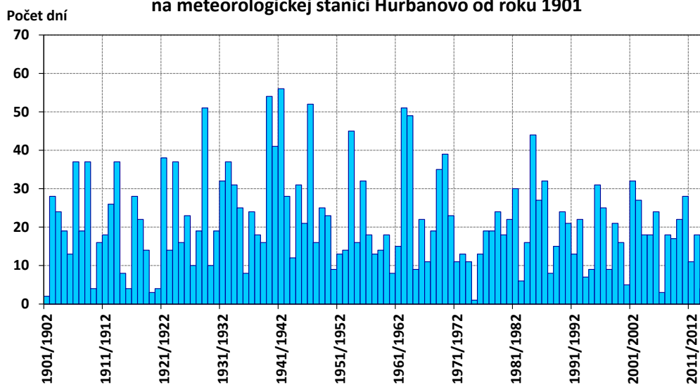
Počet ľadových dní ( T_{max} < 0\text{ }^{\circ}\text{C} ) v období (XII - II) na meteorologickej stanici Hurbanovo od roku 1901
