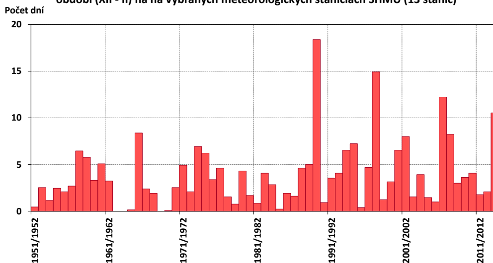
Priemerný priestorový počet dní s maximálnou teplotou vzduchu \geq 10\text{ }^{\circ}\text{C} v období (XII - II) na vybraných meteorologických staniách SHMÚ (13 staníc)
