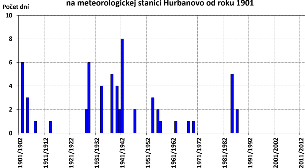
Počet arktických dní ( T_{max} \leq -10\text{ }^{\circ}\text{C} ) v období (XII - II) na meteorologickej stanici Hurbanovo od roku 1901
