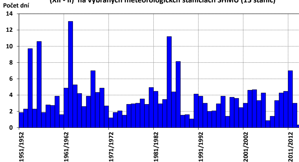
Priemerný priestorový počet arktických dní ( T_{max} \leq -10\text{ °C} ) v období (XII - II) na vybraných meteorologických stanicích SHMÚ (15 stanic)
