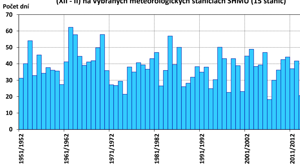
Priemerný priestorový počet ľadových dní ( T_{max} < 0\text{ }^{\circ}\text{C} ) v období (XII - II) na vybraných meteorologických staniách SHMÚ (15 staníc)
