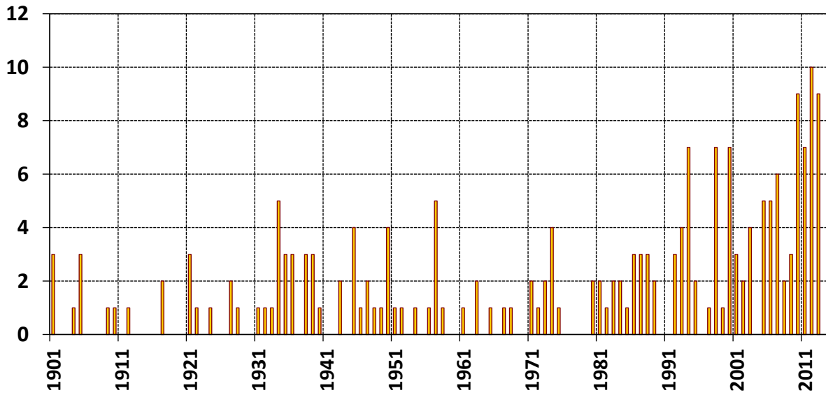
Počet tropických nocí ( T_{min} \geq 20^{\circ}\text{C} ) na meteorologickej stanici Hurbanovo v období 1901-2013
