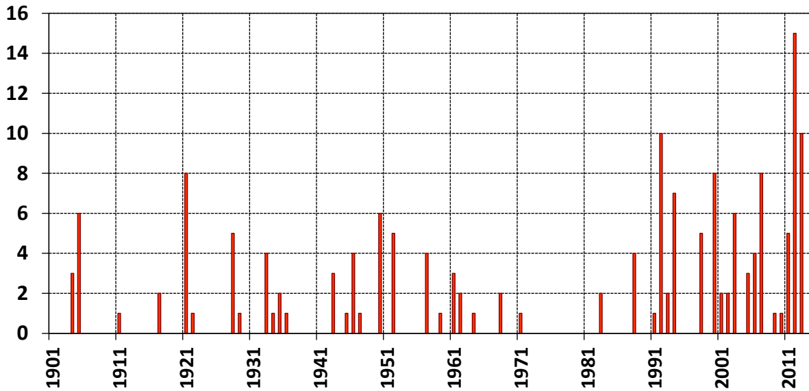
Počet supertropických dní ( T_{max} \geq 35^{\circ}\text{C} ) na meteorologickej stanici Hurbanovo v období 1901-2013
