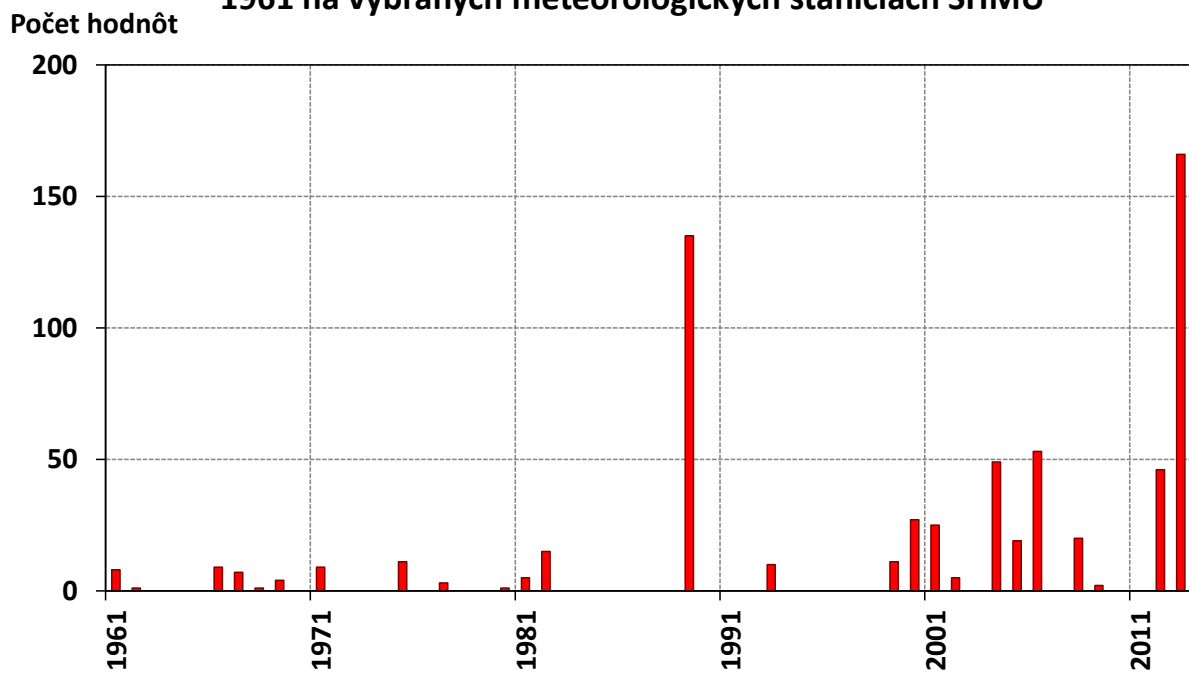
Počet hodnôt s maximálnou dennou teplotou vzduchu T_{max} \geq 20^{\circ}\text{C} v poslednej dekáde októbra (21. 10. - 31. 10.) od roku 1961 na vybraných meteorologických staniách SHMÚ
