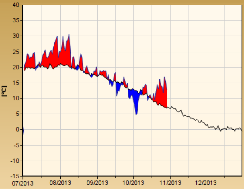
Priemerná denná teplota vzduchu - Bratislava - letisko 2013
