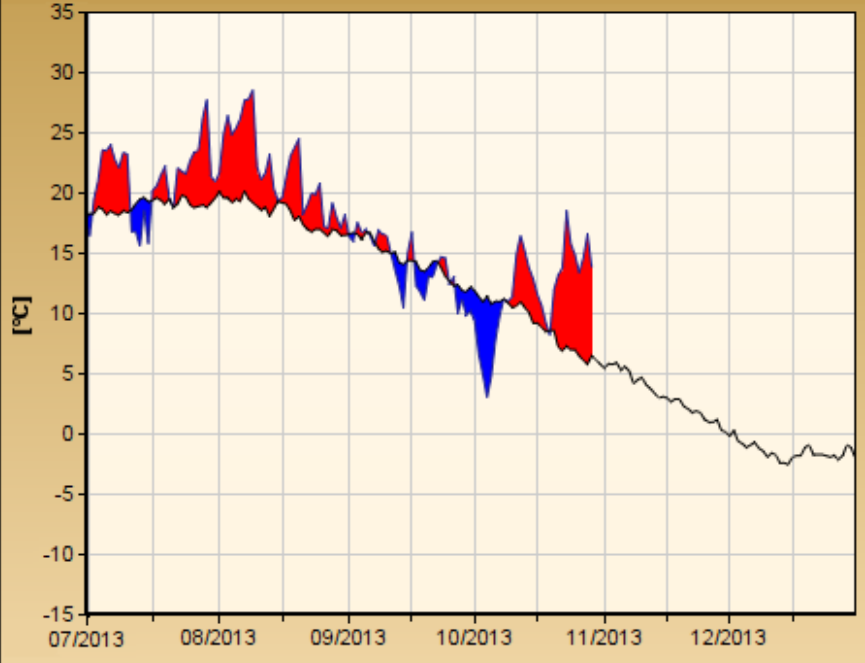
Priemerná denná teplota vzduchu - Košice - letisko 2013
