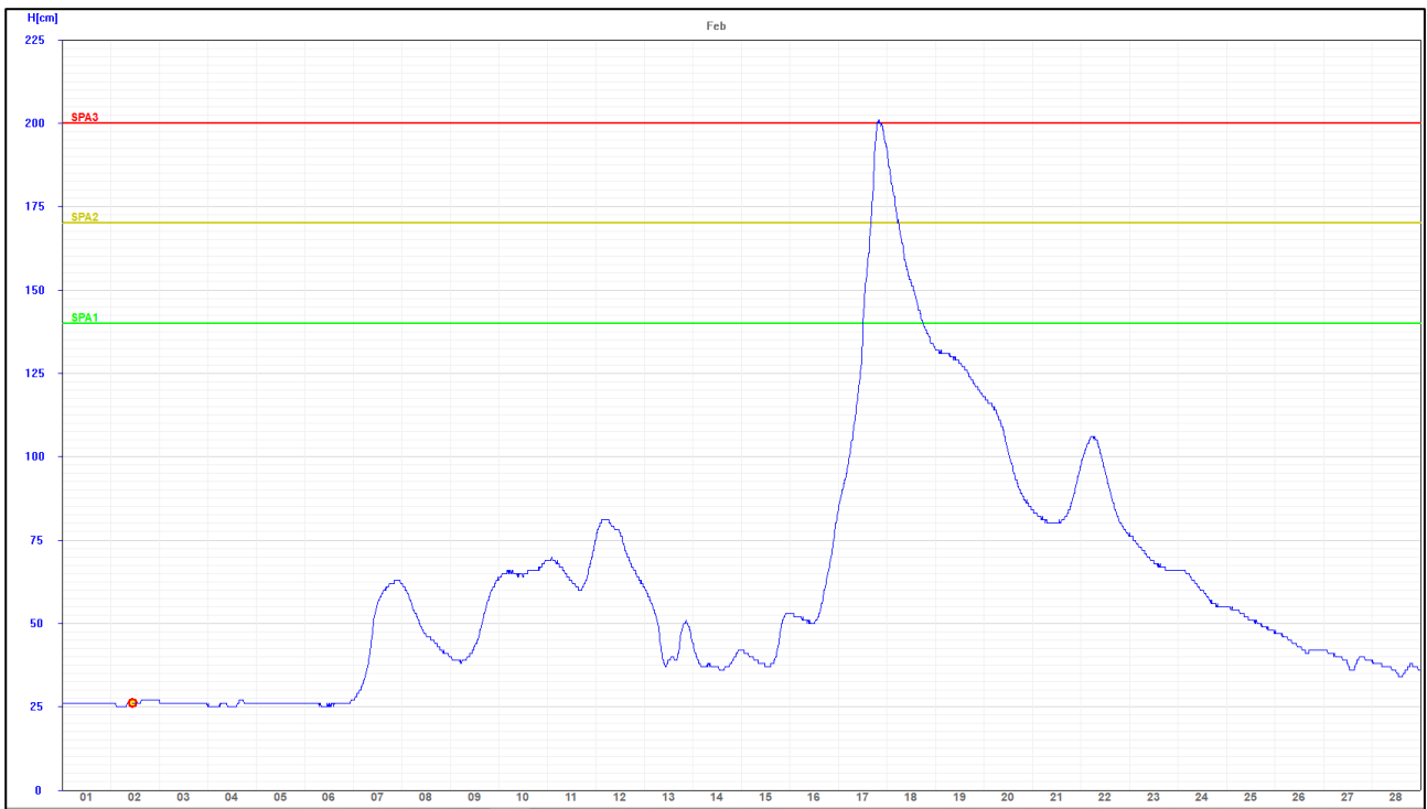
Obr. 4.3.5 Priebeh vodnej hladiny vo vodomernej stanici Ivančiná - Turiec, február 2022
