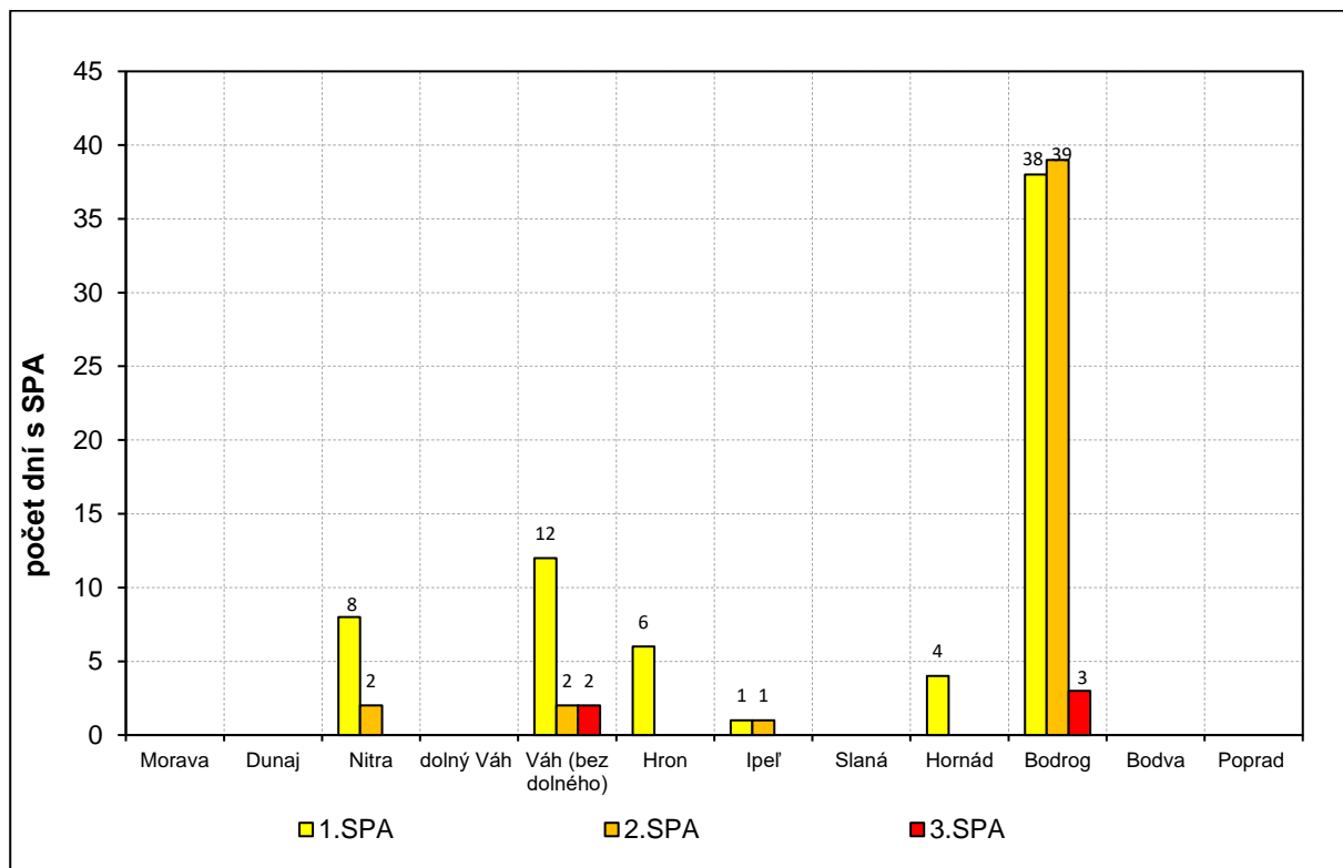
Obr. 3.1 Počet dní s SPA v jednotlivých povodiach SR v roku 2022
