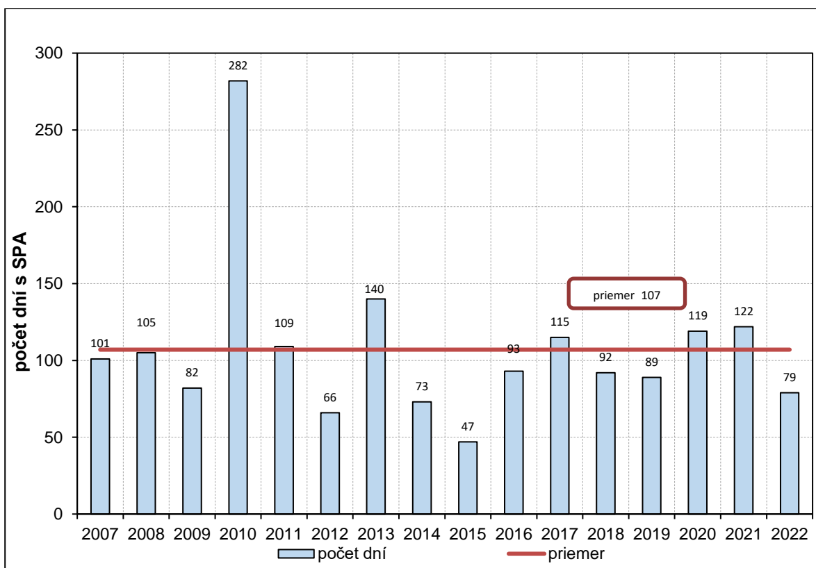
Obr. 3.4 Počet dní s SPA v operatívnych VS so stanoveným SPA od roku 2007 do roku 2022
