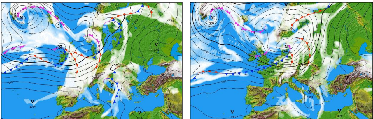
Obr. 4.3.2 Synoptická situácia v dňoch 16.2.2022 a 17.2.2022 o 0:00 UTC
