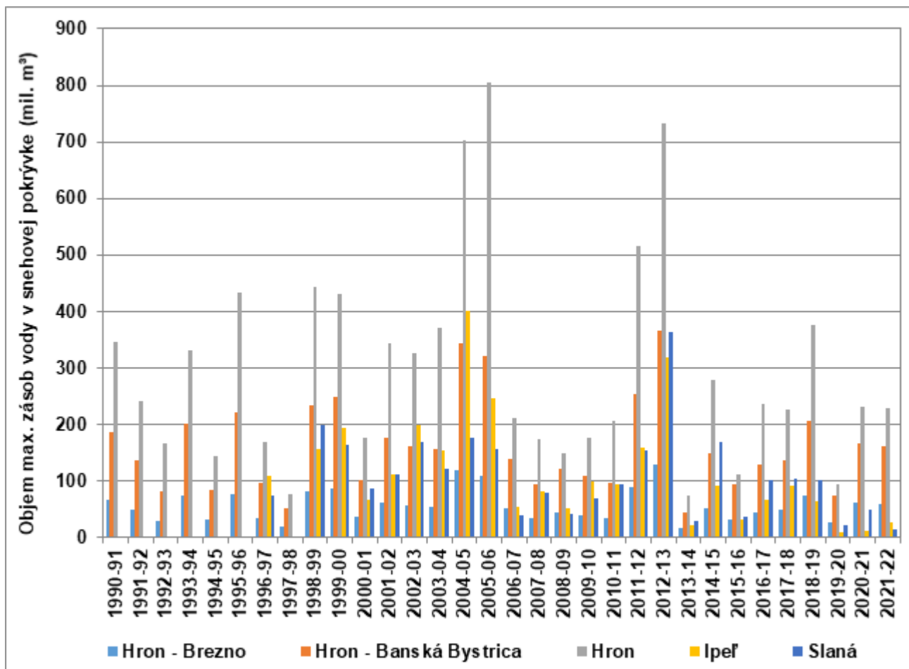
Obr. 5.2.4 Maximálne zásoby vody v snehovej pokrývke v povodí Hrona, Ipľá a Slanej od zimy 1990/1991 do zimy 2021/2022
