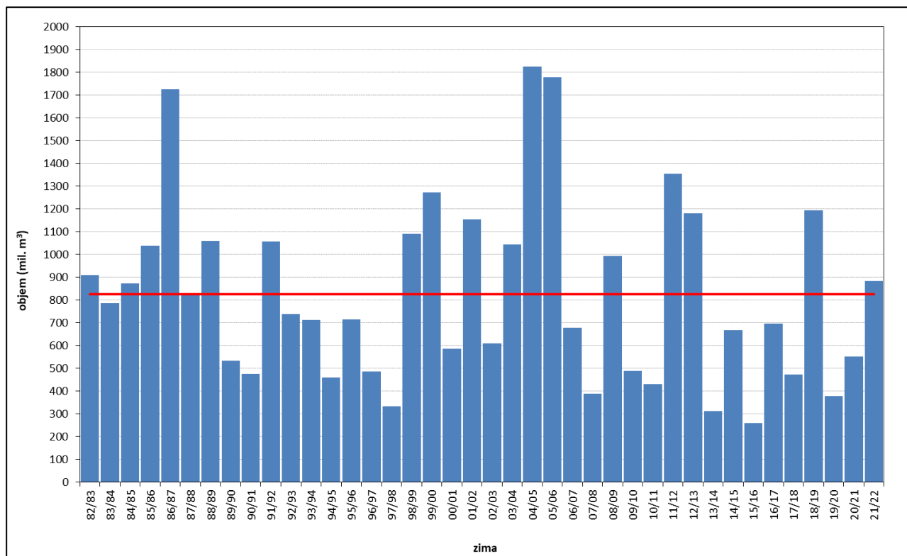
Obr. 5.1.4 Maximálne zásoby vody v snehovej pokrývke (mil. m 3 ) v povodí Váhu po profil VD Nosice a priemerná hodnota (červená čiara) 1982/83 až 2021/2022
