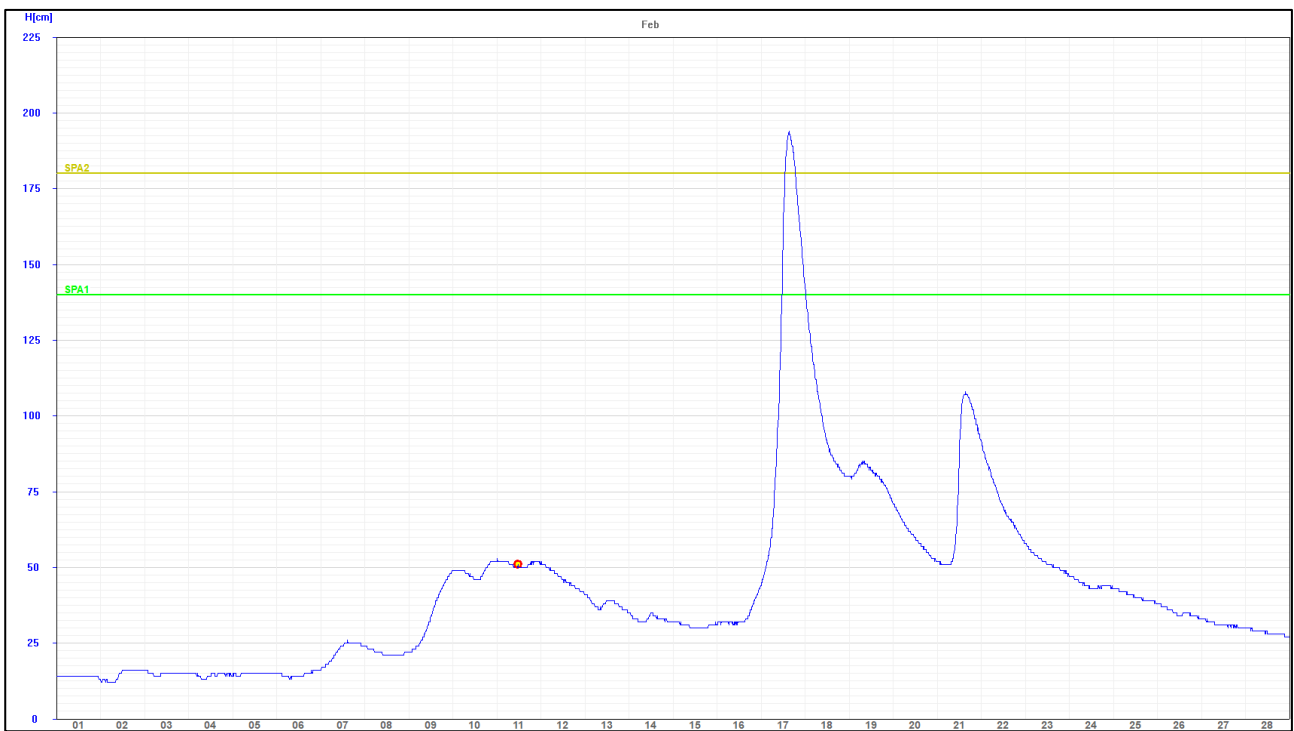
Obr. 4.3.6 Priebeh vodnej hladiny vo vodomernej stanici Čadca - Kysuca, február 2022
