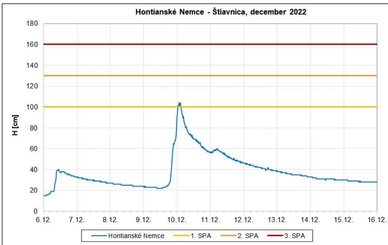
Obr. 4.6.5 Priebek vodnej hladiny vo vodomernej stanici Hontianske Nemce - Štiavnica, december 2022
