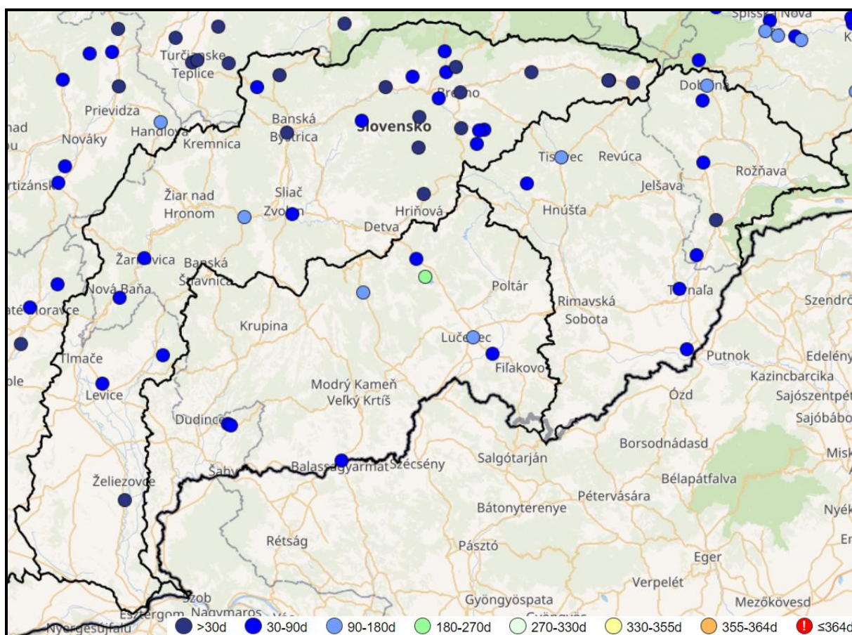
Obr. 3.7 M-dennosť priemerných denných prietokov dňa 10. 2. 2024
