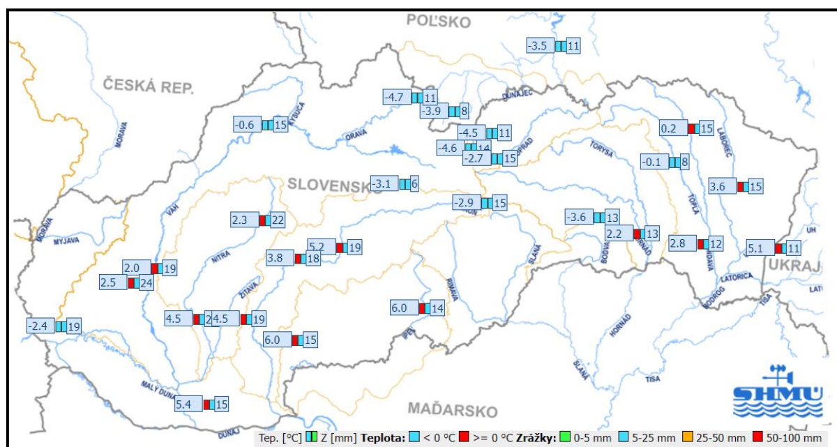
Obr. 3.2 Teplota vzduchu a 24-hodinový úhrn zrážok na Slovensku dňa 7.1. k 6:00 SEČ
