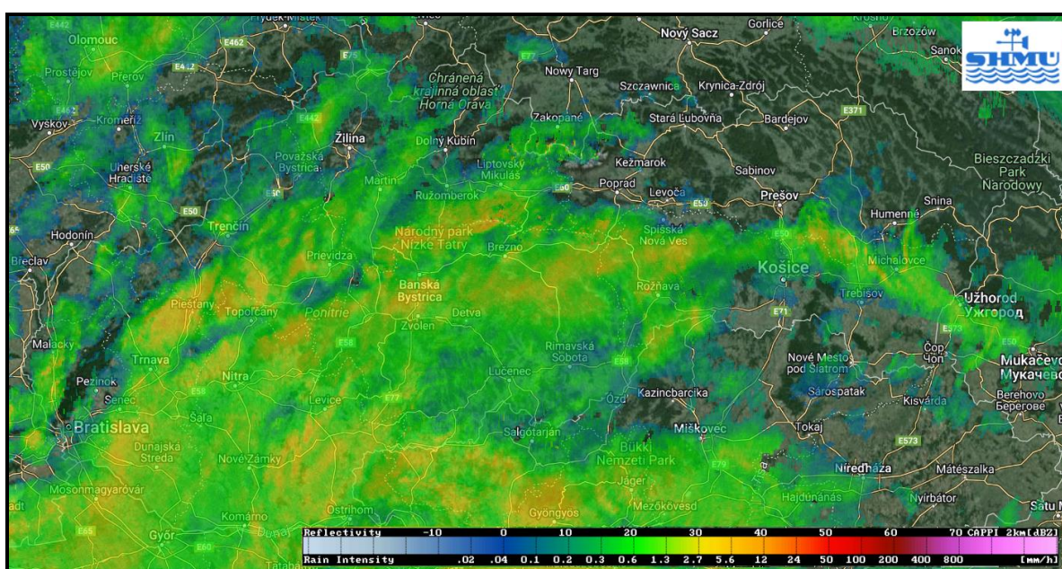
Obr. 3.6 Zrážkové pole sa zachytávalo najmä na pohoriach stredného Slovenska (11.2.2024 o 7:35 SEČ)
