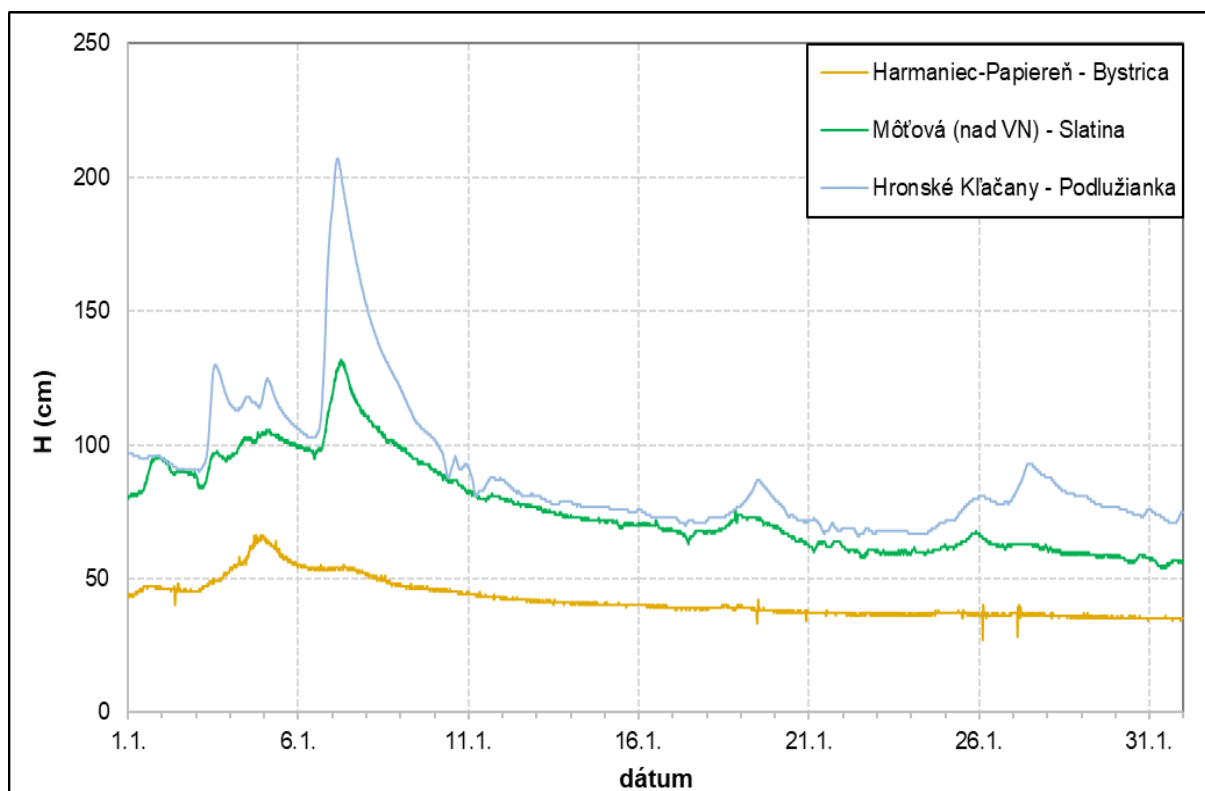
Obr. 3.4 Priebeh vodných hladín na prítokoch Hrona, január 2024
