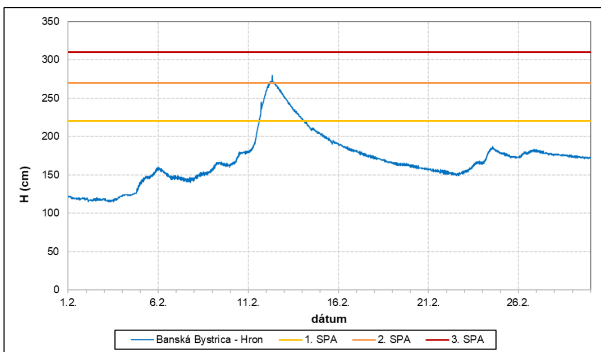
Obr. 3.9 Pribeh vodnej hladiny vo vodomernej stanici Banská Bystrica – Hron, február 2024
