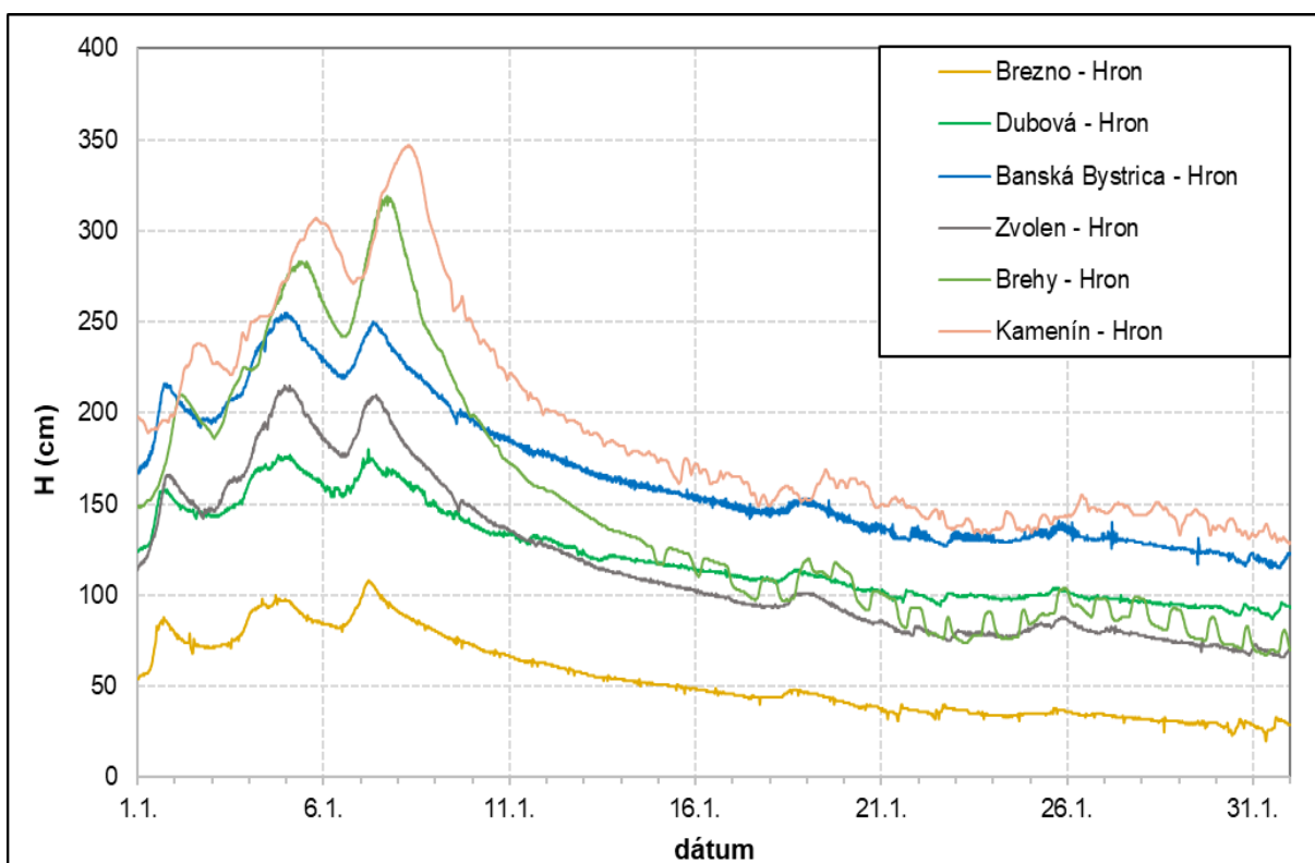
Obr. 3.5 Priebeh vodných hladín vo vodomerných staniciach na Hrone, január 2024
