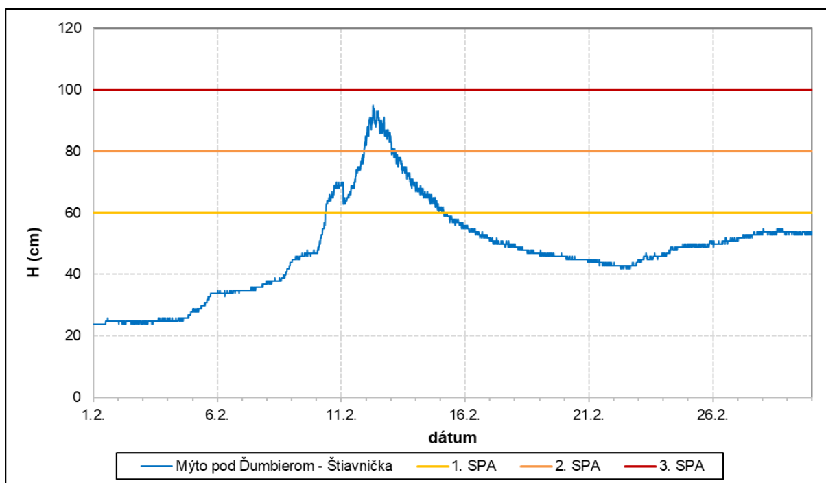
Obr. 3.8 Pribeh vodnej hladiny vo vodomernej stanici Mýto pod Ďumbierom – Štiavnička, február 2024
