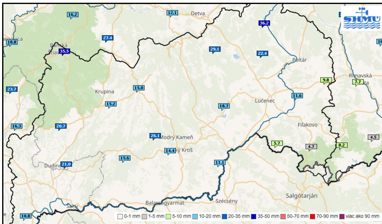
Obr. 3.13 24-hodinové úhrny zrážok v povodí Ipľa 12.2.2024 k 0:00 SEČ
