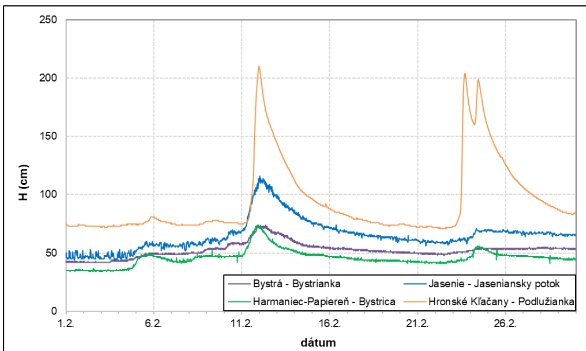
Obr. 3.10 Pribeh vodných hladín na tokoch v povodí Hrona, február 2024
