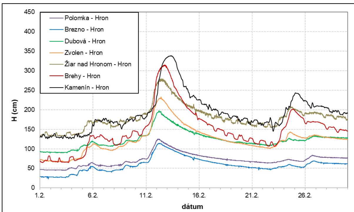
Obr. 3.11 Pribeh vodných hladín vo vodomerných staniciach na Hrone, február 2024
