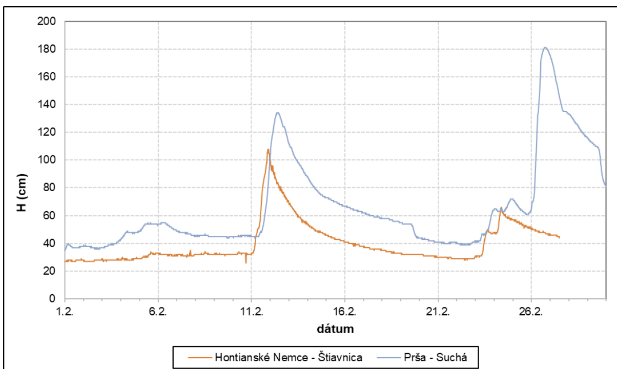
Obr. 3.15 Priebeh vodných hladín na tokoch v povodí Ipľa, február 2024
