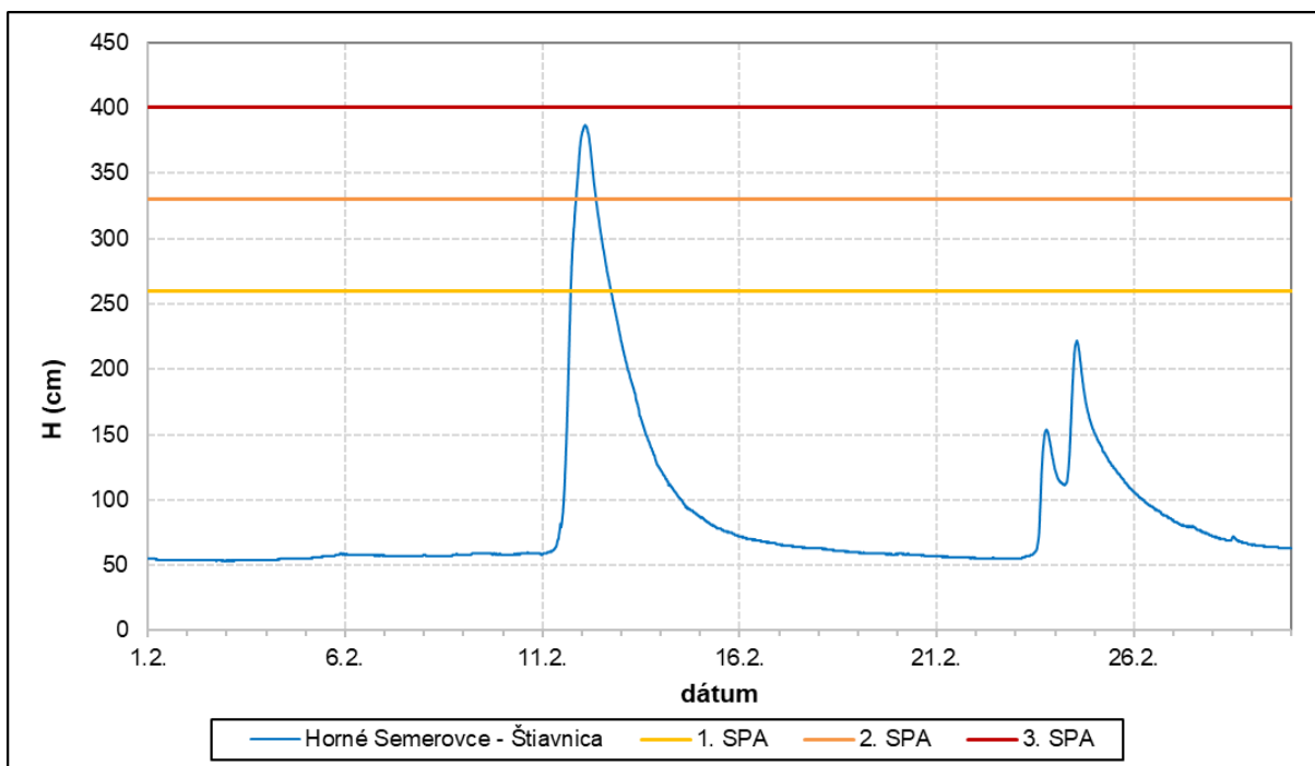
Obr. 3.14 Priebeh vodnej hladiny vo vodomernej stanici Horné Semerovce – Štiavnica, február 2024
