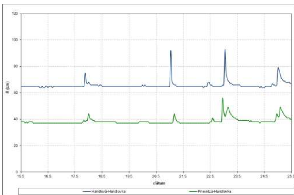
Obr. 4.4.7 Pribeh vodných hladín na Handlovke, máj 2024
