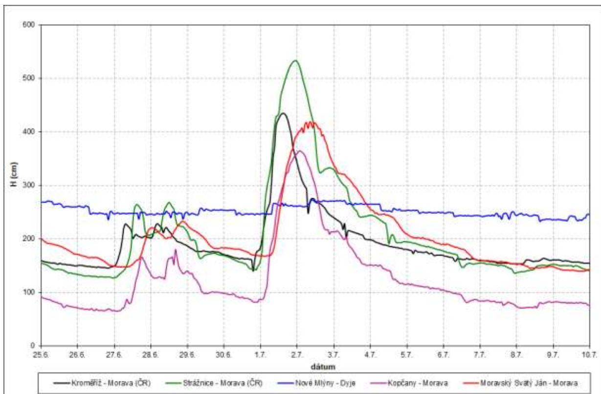
Obr. 4.1.6 Priebek vodných hladín na tokoch v povodí Moravy na jej českom a slovenskom úseku, jún – júl 2024
