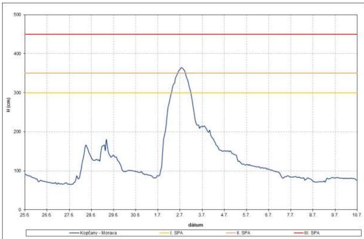
Obr. 4.1.5 Priebek vodnej hladiny vo vodomernej stanici Kopčany – Morava, jún – júl 2024
