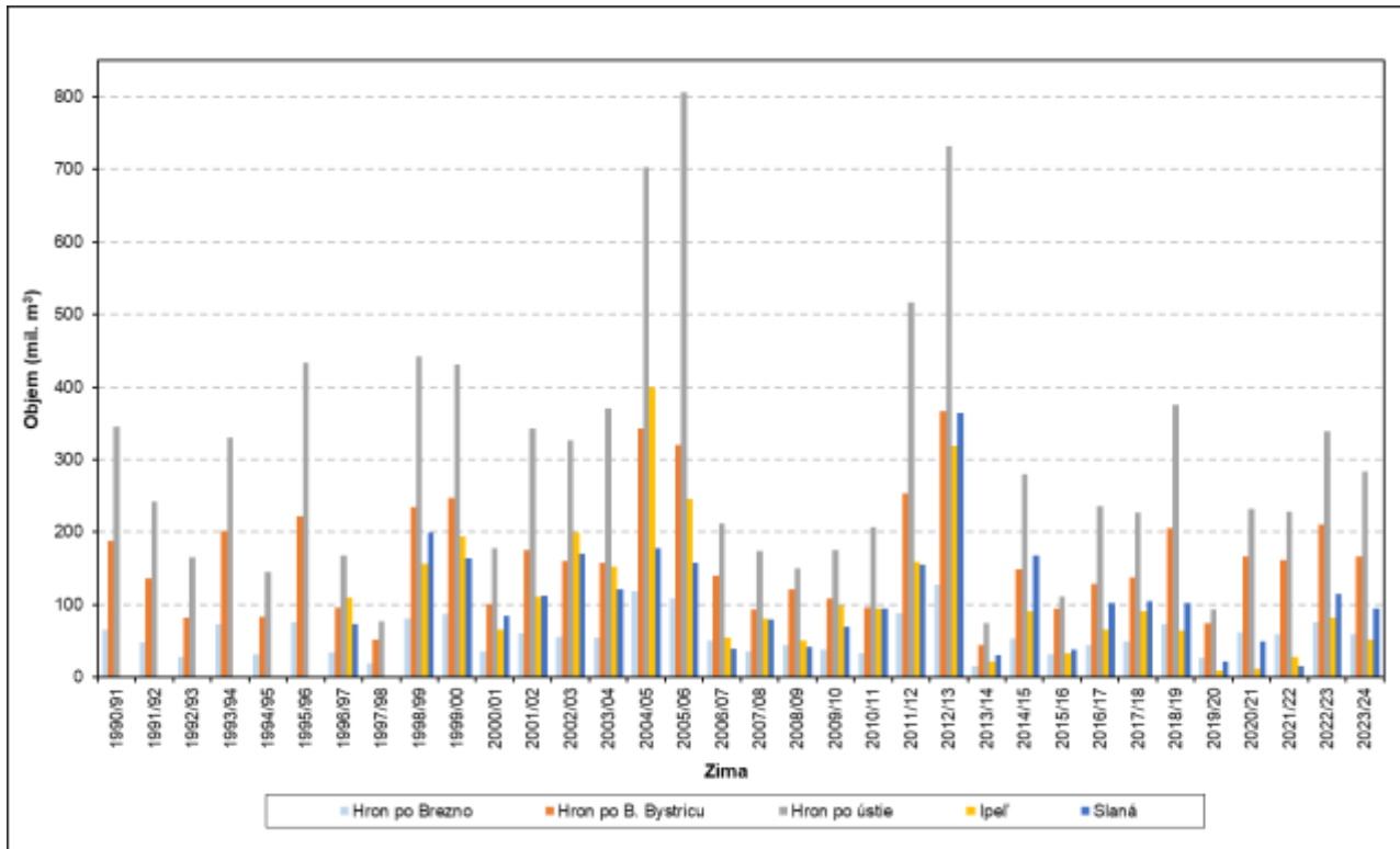
Obr. 5.3.2 Maximálne zásoby vody v snehovej pokrývke v povodí Hrona, Ipľa a Slanej v období 1990/1991 až 2023/2024
