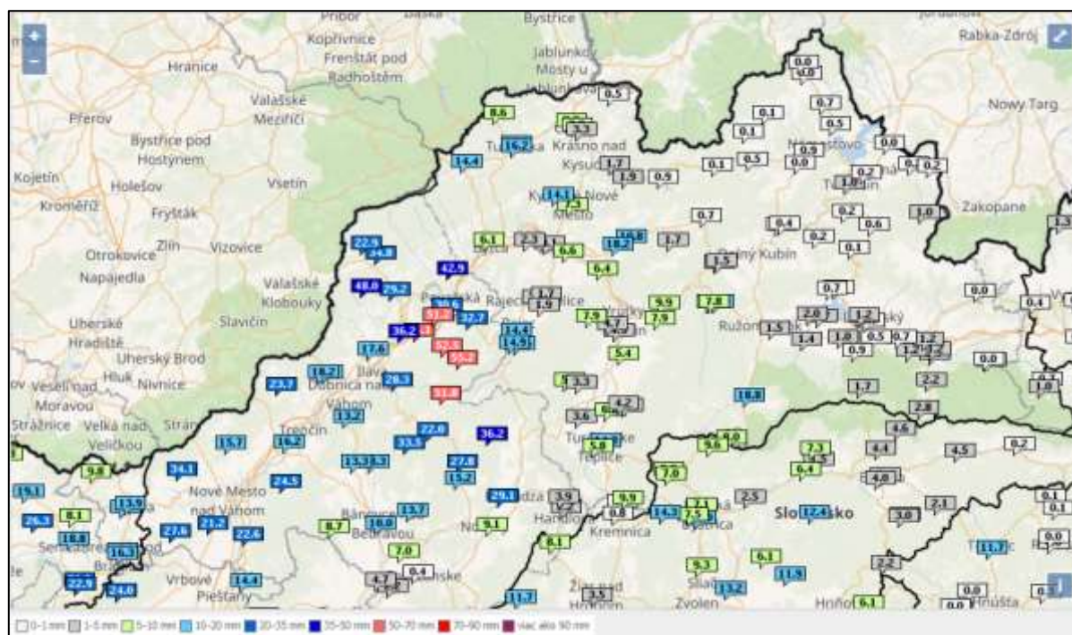
Obr. 4.3.8 Úhrn atmosférických zrážok za predchádzajúcich 24 hodín v povodí horného a stredného Váhu dňa 27.6.2024 k 6:00 hod.
