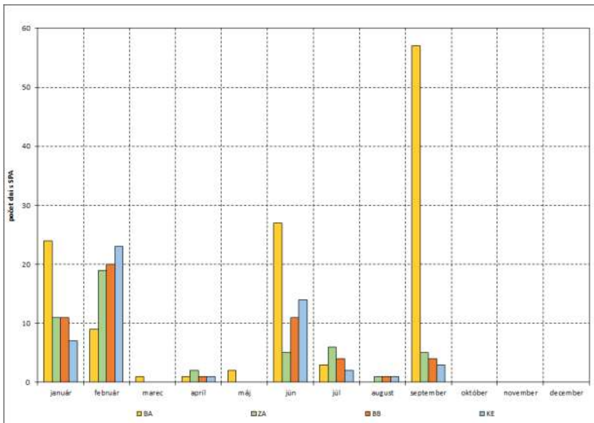
Obr. 3.2 Počet dní s SPA v jednotlivých mesiacoch roka 2024 v operatívnych VS (SR) podľa regionálnych pracovísk
