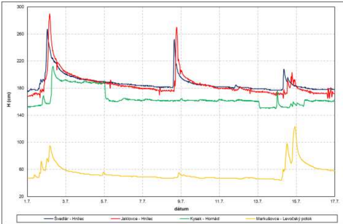
Obr. 4.9.10 Priebeh vodných hladín v povodí Hornádu, júl 2024
