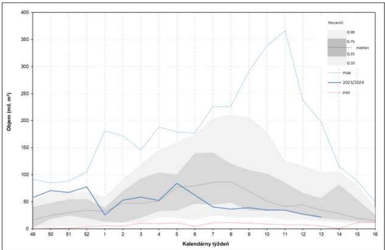
Obr. 5.4.3 Priebeh celkových zásob vody v snehovej pokrývke (mil. m 3 ) v povodí Popradu počas zimy 2023/2024 v štatistickom porovnaní s ostatnými zimami od 2004/2005
