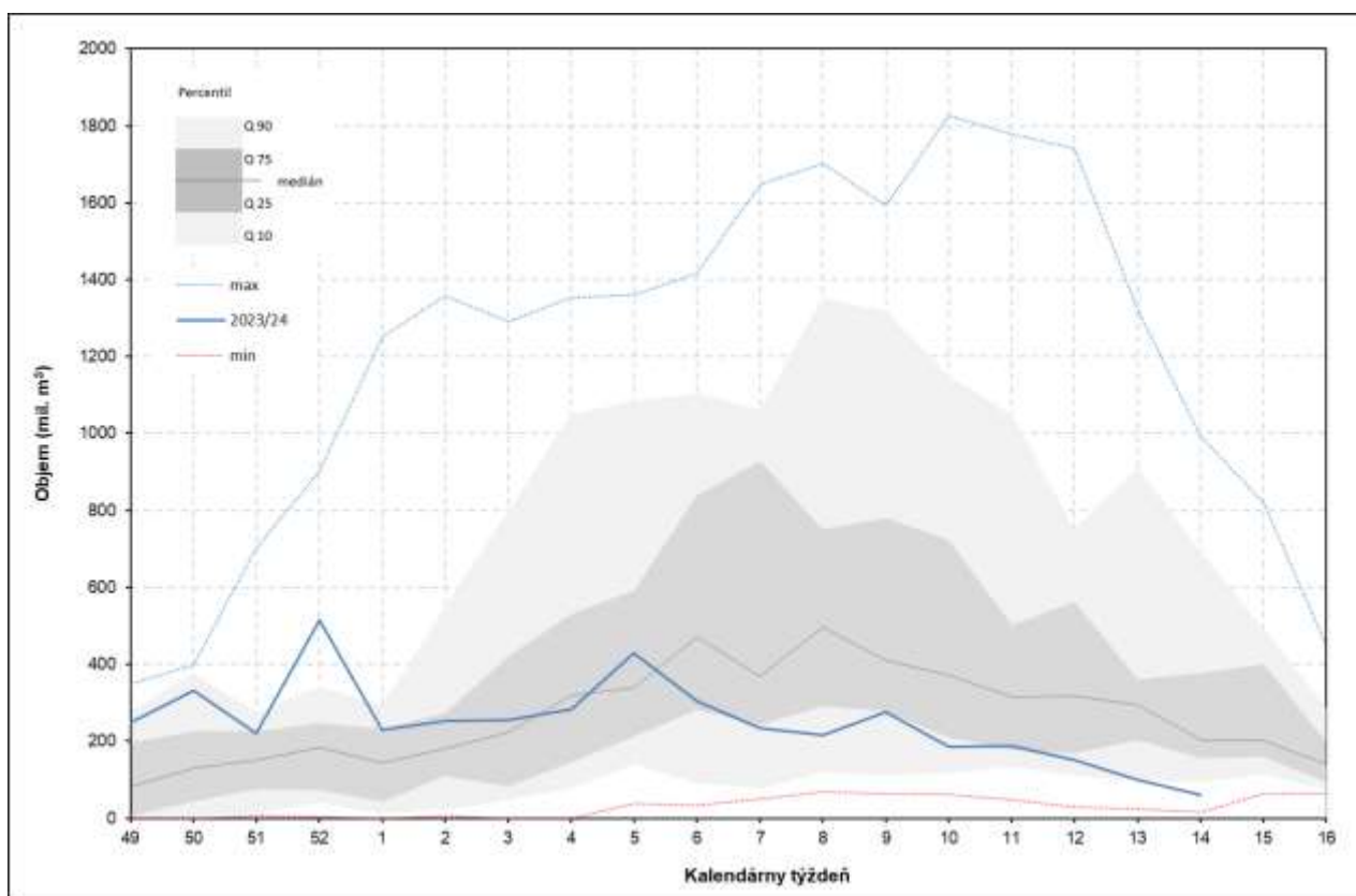
Obr. 5.2.3 Priebeh celkových zásob vody v snehovej pokrývke (mil. m 3 ) v povodí Váhu po profil VD Nosice počas zimy 2023/2024 v štatistickom porovnaní s ostatnými zimami od 2004/2005
