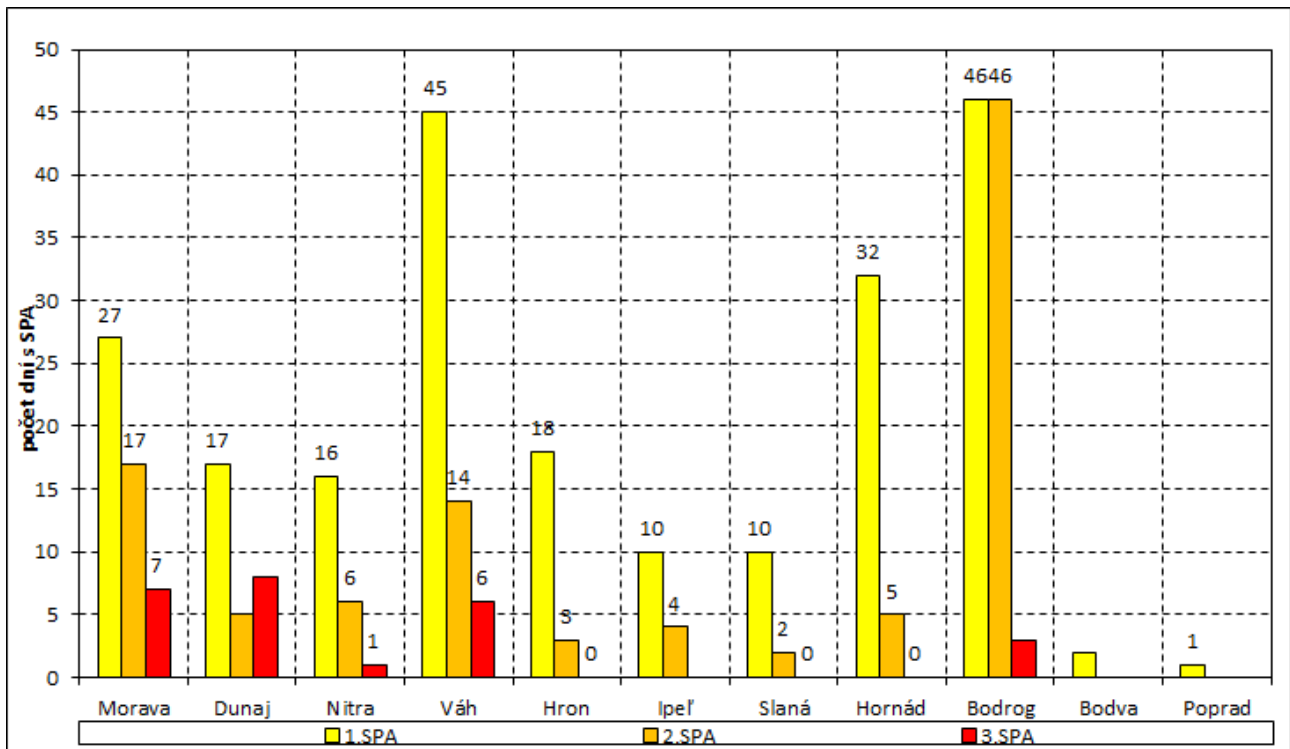
Obr. 3.1 Počet dní s SPA v jednotlivých povodiach SR v roku 2024
