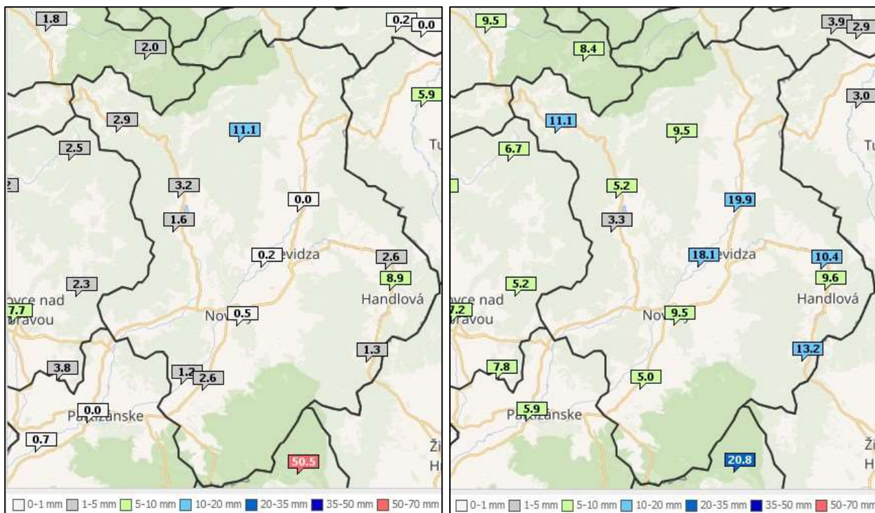
Obr. 4.4.6 Úhrn atmosférických zrážok za predchádzajúcich 24 hodín na povodie Nity, dňa 21.5.2024 o 6:00 hod. (vľavo) a 23.5.2024 o 6:00 hod. (vpravo)
