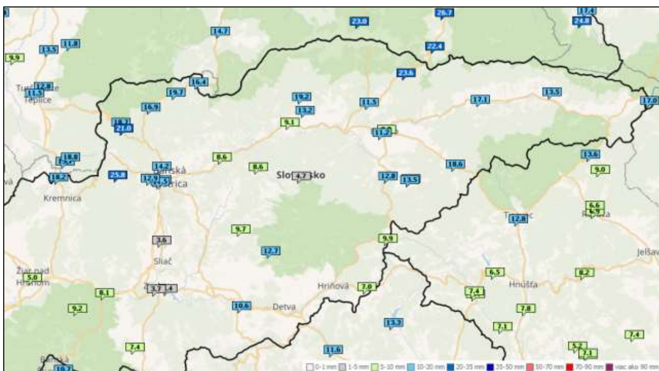
Obr. 4.5.3 Úhrn atmosférických zrážok za predchádzajúcich 24 hodín (mm) dňa 3.4.2024 o 06:00 hod.
