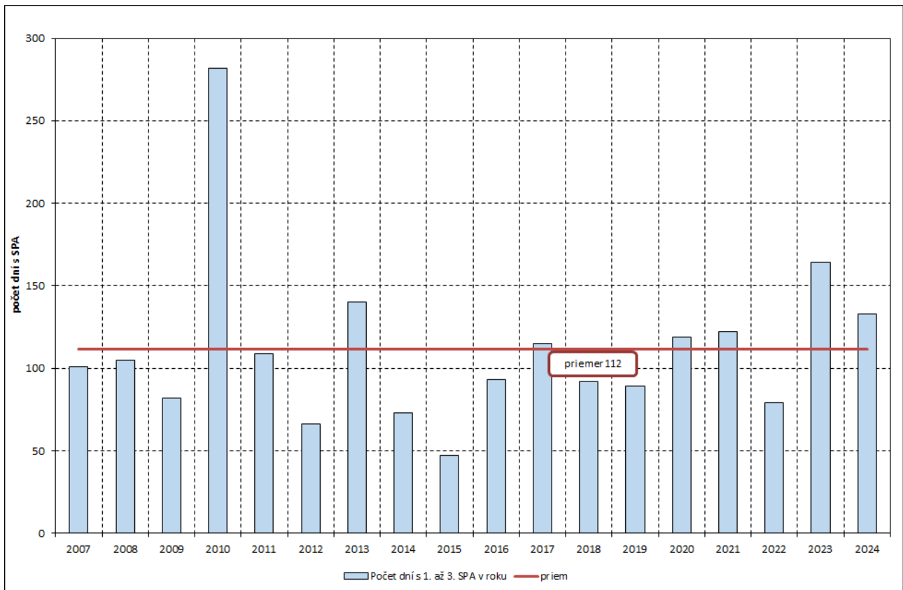
Obr. 3.4 Počet dní s SPA vo operatívnych VS so stanoveným SPA od roku 2007 do 2024
