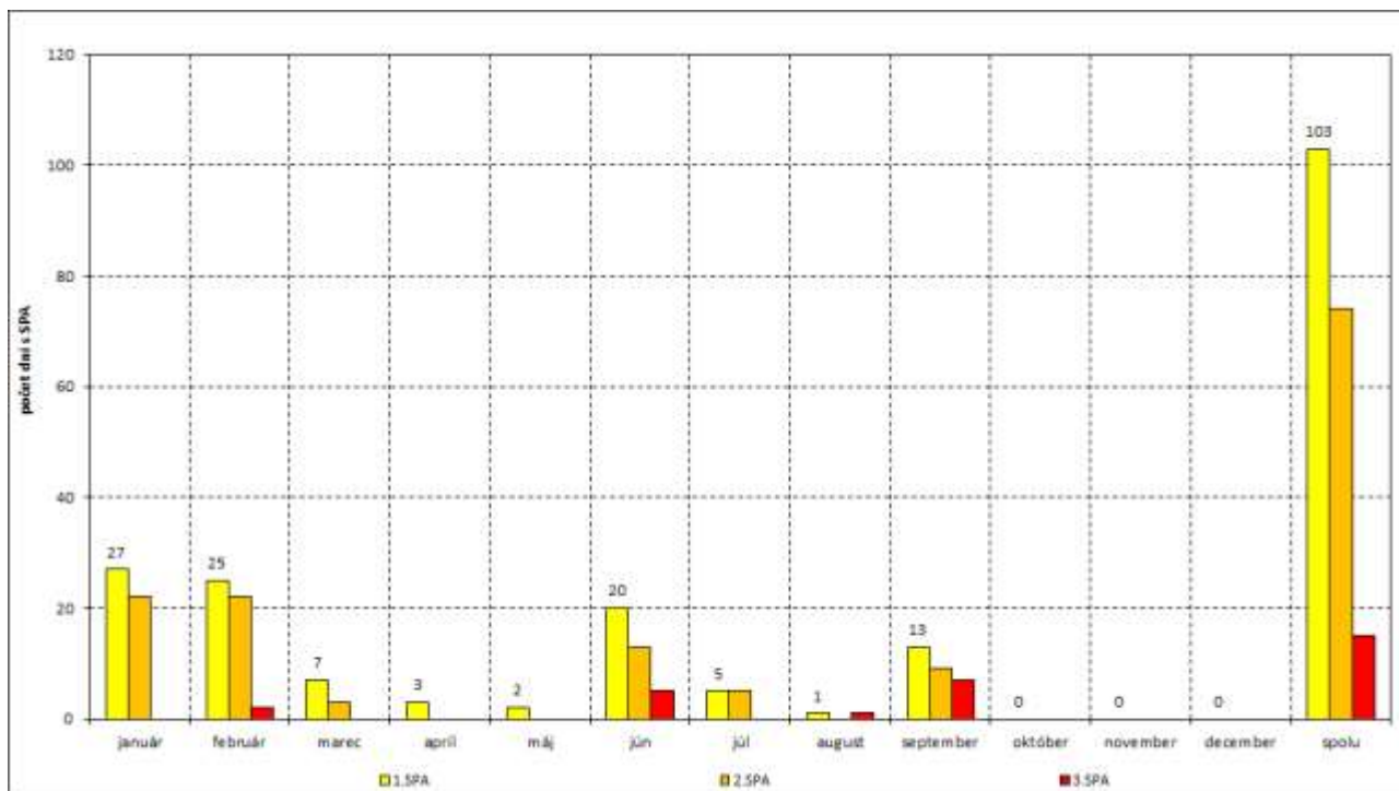
Obr. 3.3 Počet dní s SPA v jednotlivých mesiacoch roka 2024 v operatívnych VS (SR)
