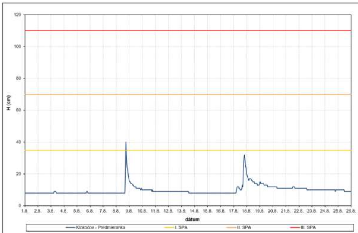
Obr. 4.3.21 Priebeh vodných hladín vo vodomernej stanici Klokočov – Predmieranka, august 2024
