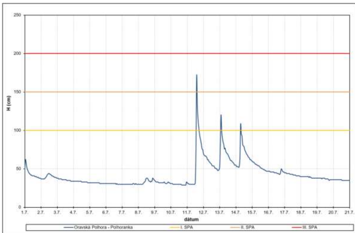
Obr. 4.3.15 Priebeh vodnej hladiny vo vodomernej stanici Oravská Polhora – Polhoranka, júl 2024
