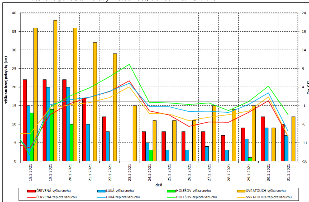
Obr. 3.1 Výška snehovej pokrývky a teplota vzduchu vo vybraných synoptických staniciach českého povodia Moravy k 6:00 hod., v dňoch 18. - 31.1.2021
