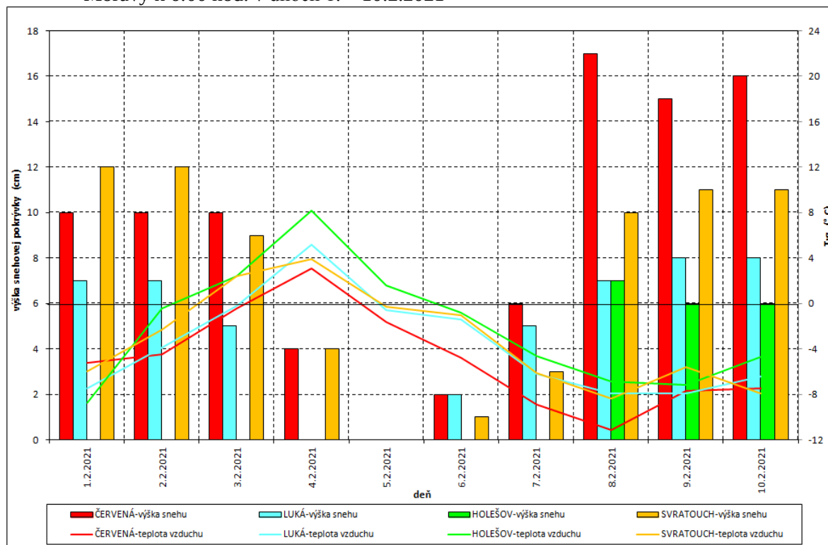
Obr. 3.4 Výška snehovej pokrývky a teplota vzduchu vo vybraných staniciach českého povodia Moravy k 6:00 hod. v dňoch 1. – 10.2.2021
