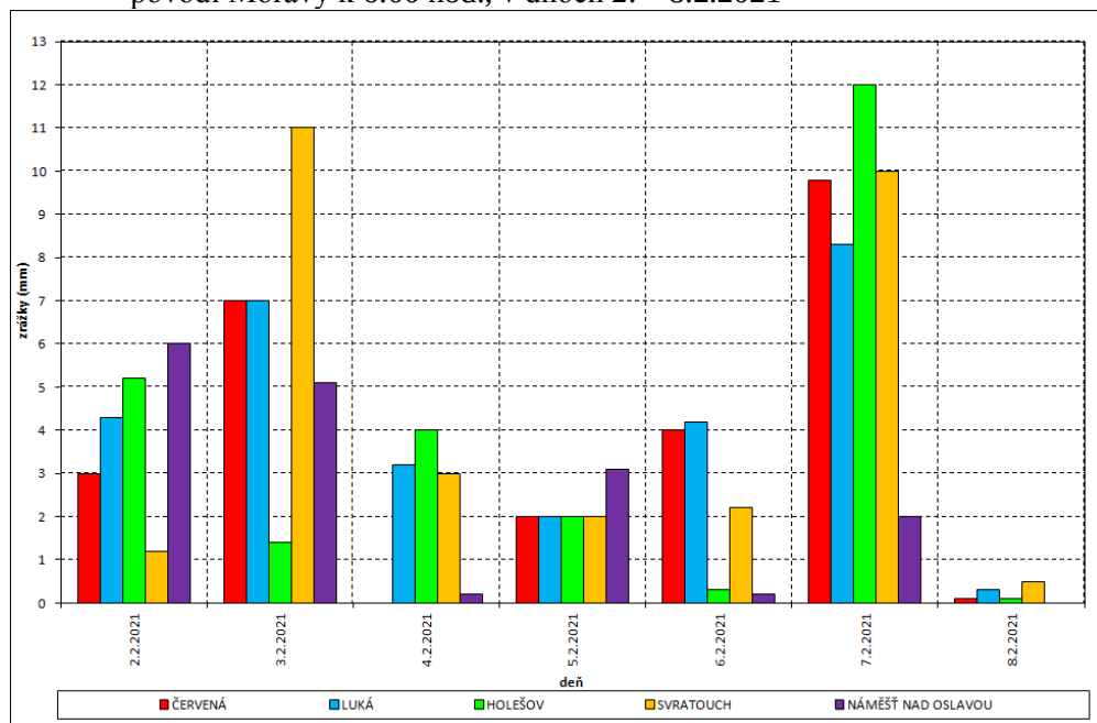
Obr. 3.5 24-hod. úhrny zrážek vo vybraných zrážkomerných staniách v českém povodí Moravy k 6:00 hod., v dnech 2. – 8.2.2021
