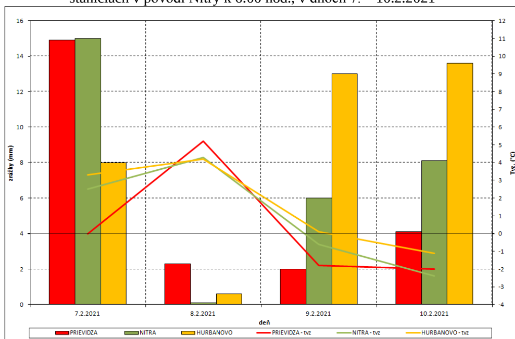
Obr. 3.13 24-hod. úhrny zrážok a teplota vzduchu vo vybraných synoptických staniciach v povodí Nitry k 6:00 hod., v dňoch 7. - 10.2.2021
