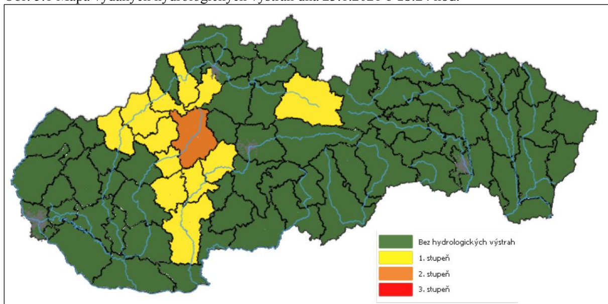
Obr. 5.1 Mapa vydaných hydrologických výstrah dňa 23.1.2021 o 18:24 hod.
