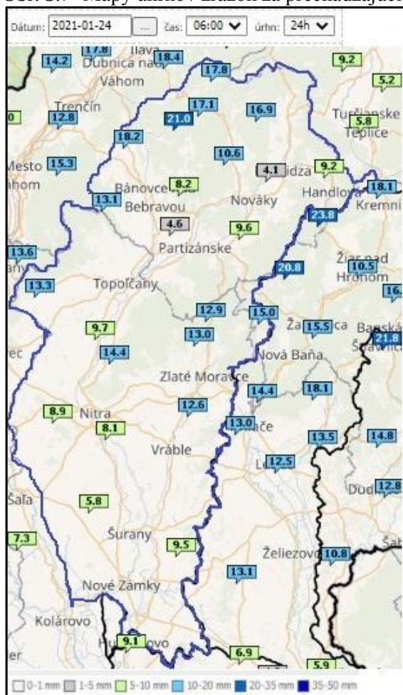
Obr. 3.7 Mapy úhrnov zrážok za prechádzajúcich 24 hod. v povodí Nitry, namerané dňa 24.1.2021 a 8.2.2021
