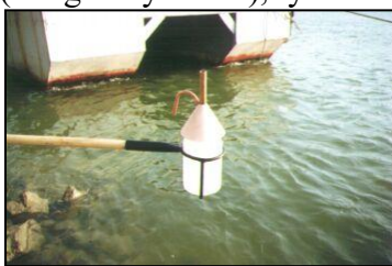
Obrázok 3 Vzorkovač.
