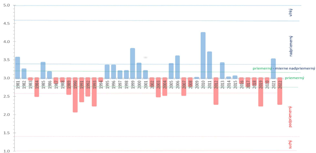
Obr. 9 Zhodnotenie jednotlivých rokov obdobia 1981 – 2022 z hľadiska podzemnej vody
