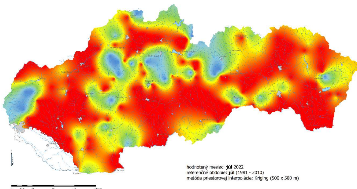
Obr. 5 Priestorové hodnotenie podzemnej vody v júli 2022
