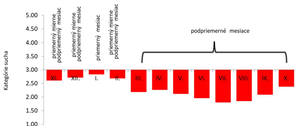
Obr. 7 Hodnotenie jednotlivých mesiacov hydrologického roka 2022 z pohľadu podzemnej vody
