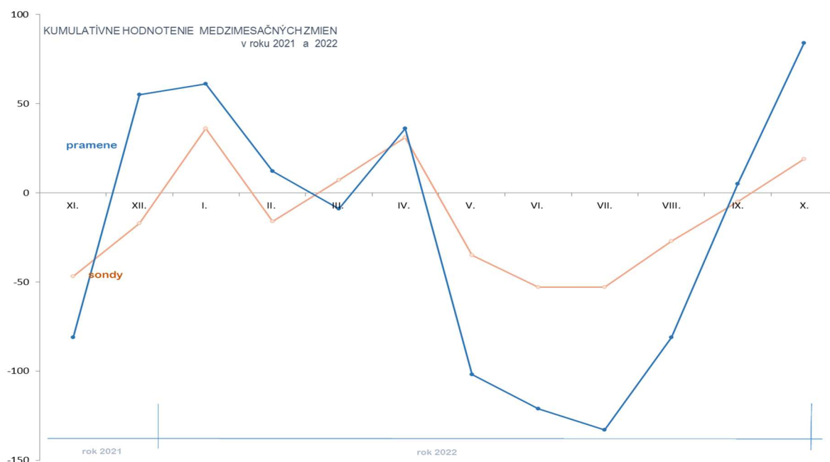
Obr. 6 Kumulatívne zobrazenie medzimesačných zmien v objektoch podzemnej vody (nárasty/poklesy hladiny podzemnej vody, resp. výdatností prameňov) v hydrologickom roku 2022
