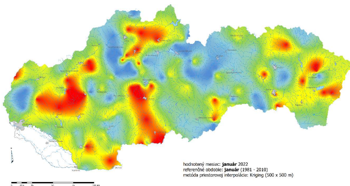
Obr. 4 Priestorové hodnotenie podzemnej vody v januári 2022
