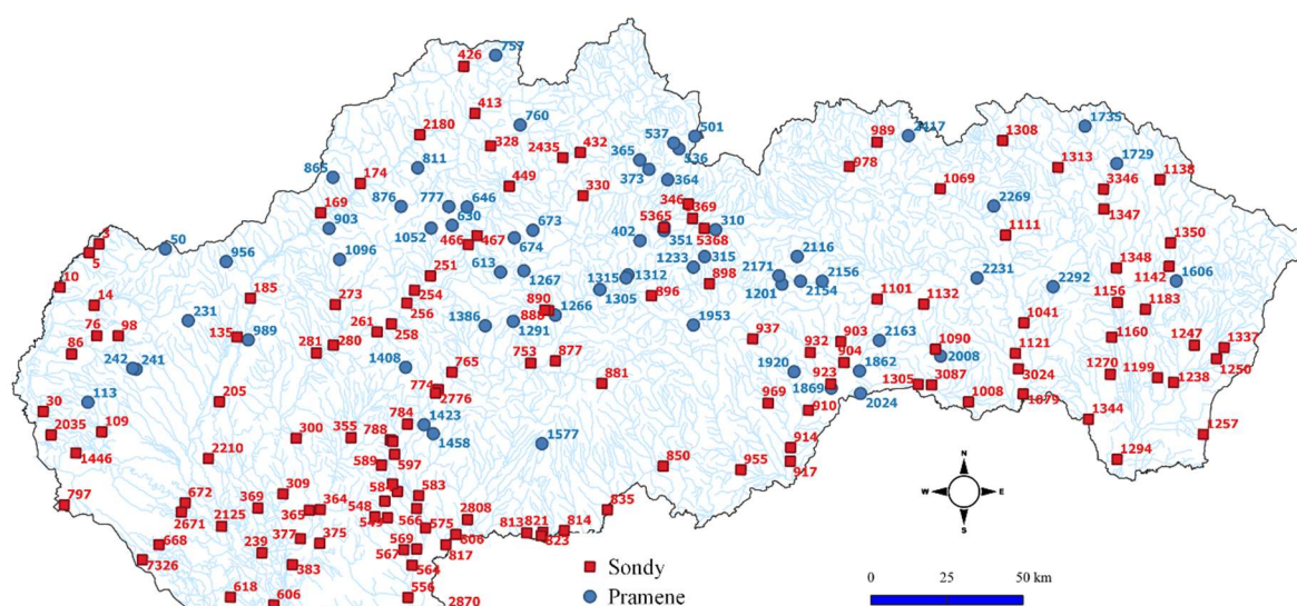
Obr. 1 Lokalizácia hodnotených objektov
