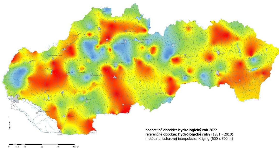
Obr. 8 Priestorové hodnotenie podzemnej vody v hydrologickom roku 2022
